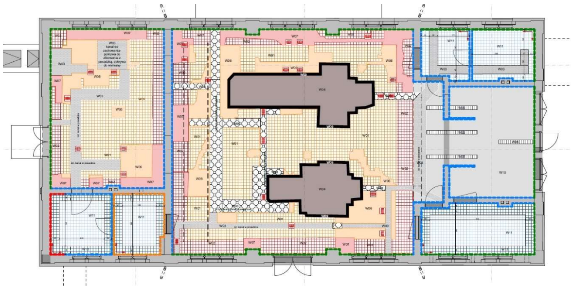
Ryc. 3. Projekt wykończenia posadzek i ścian budynku elektrowni na Westerplatte
