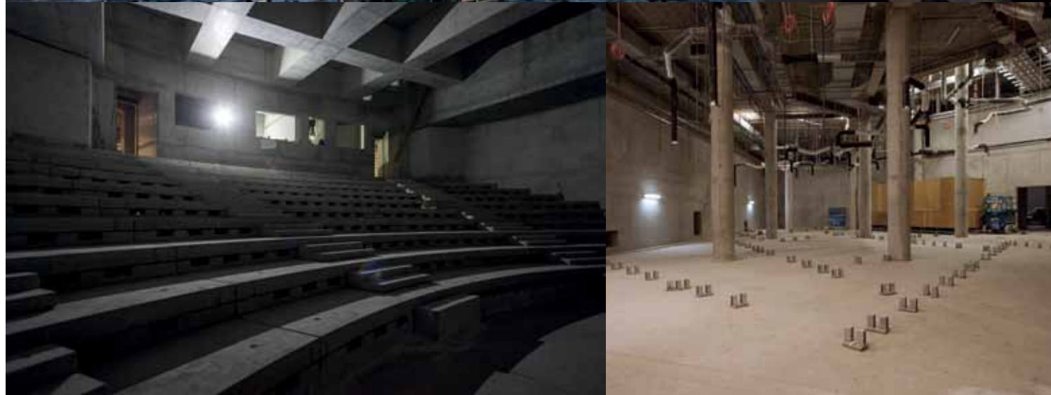
U góry z prawej: najwyższy punkt konstrukcyjny wieży. Na dole z lewej: stan surowy sali konferencyjnej, z prawej: przestrzeń jednej z sal wystawowych. Fot. Roman Jocher
